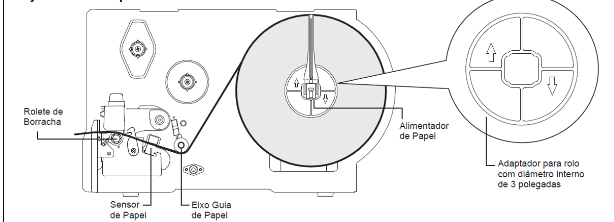
Fig.9 –Diagrama de instalação do rolo de etiquetas
