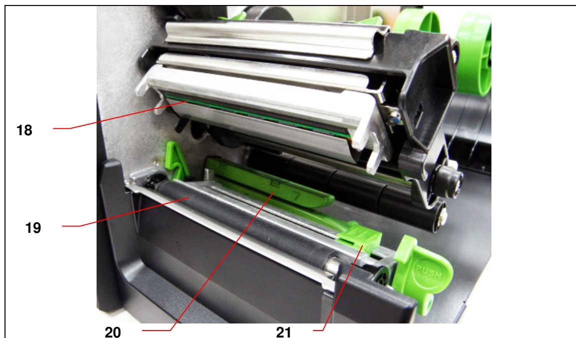
Fig.4 - Vista do mecanismo de impressão
