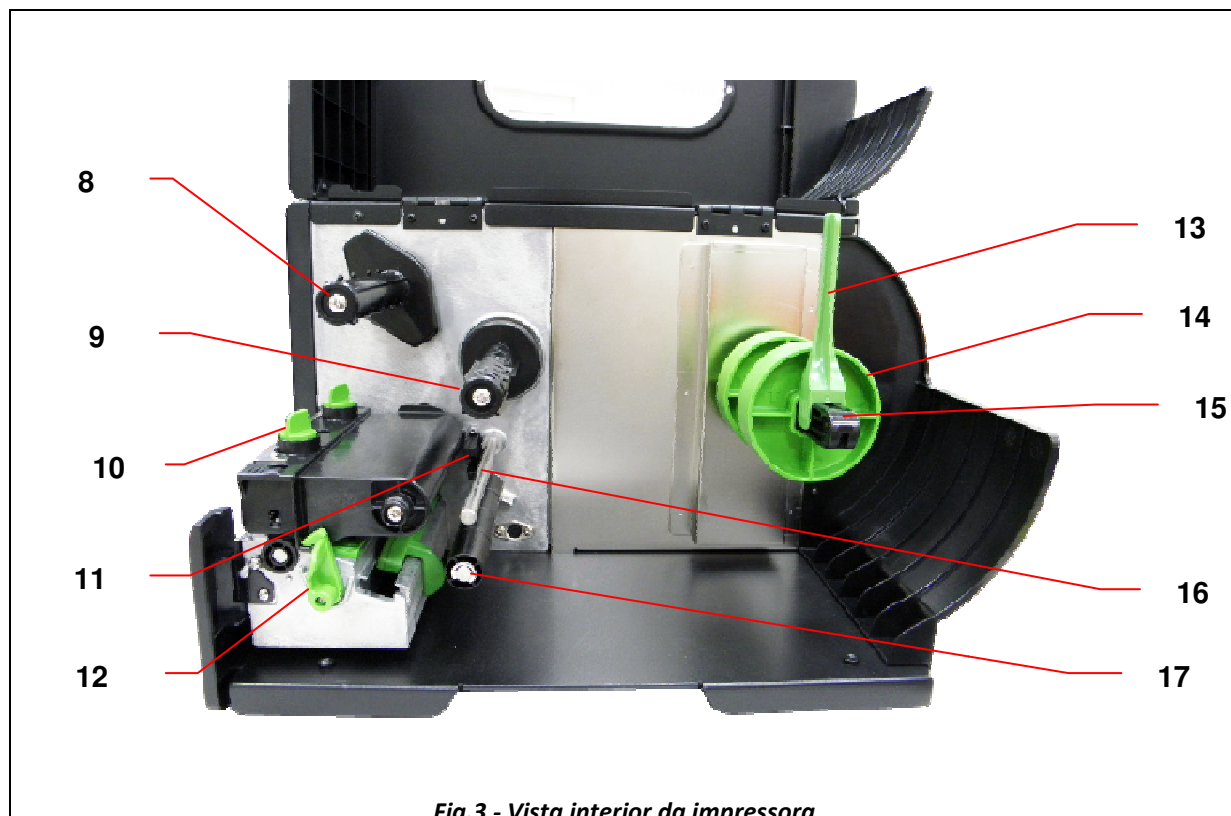
Fig.3 - Vista interior da impressora
